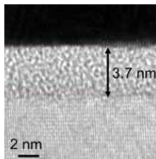
Ultradünne Neodymoxidschicht auf Siliziumwafer
